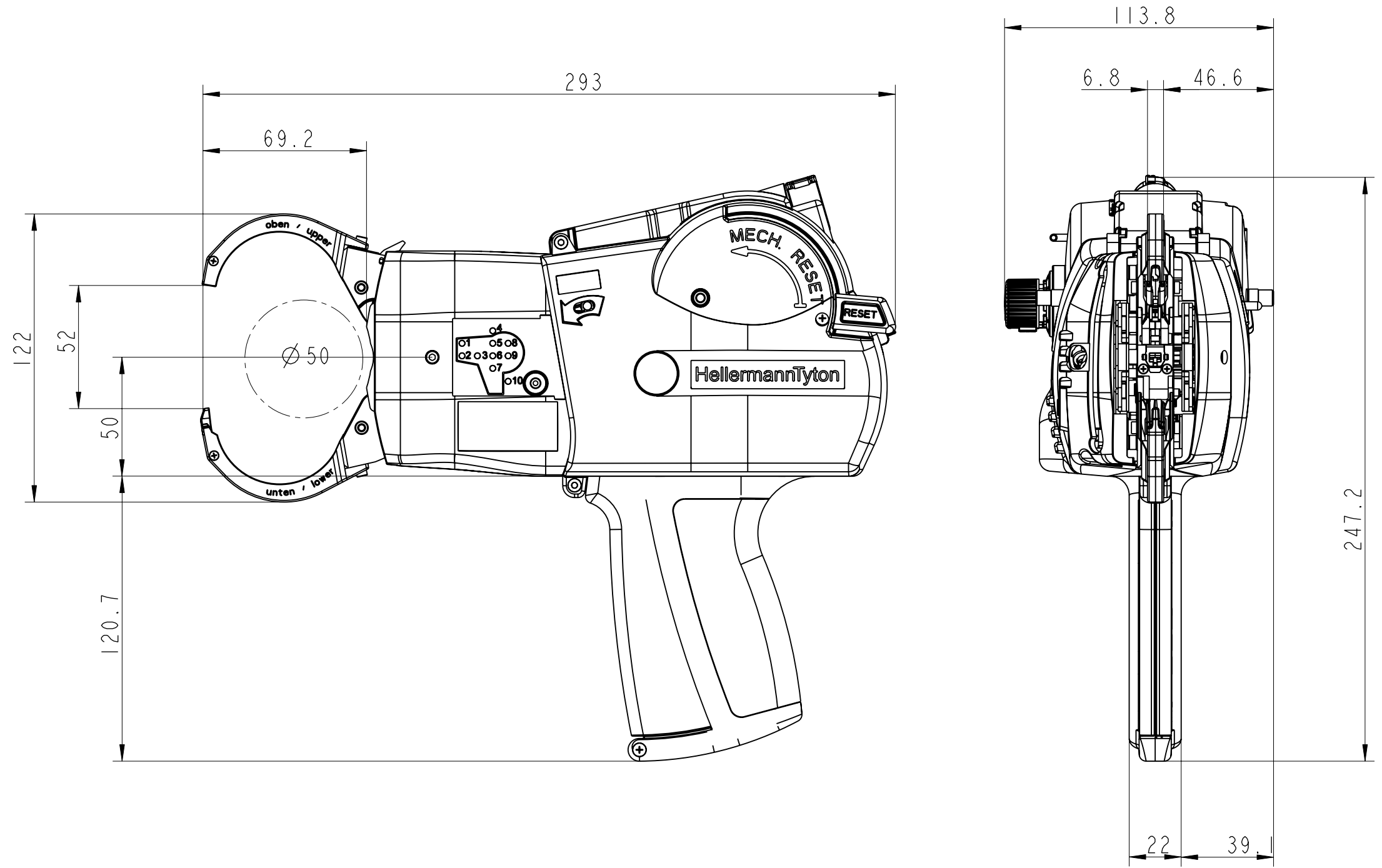
ATS3080 Hauptabmessungen
