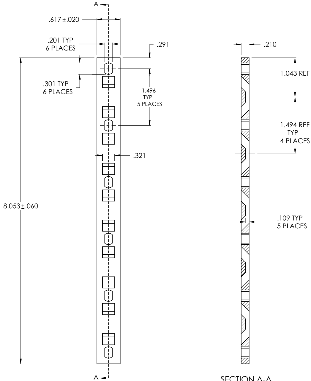
SECTION A-A
